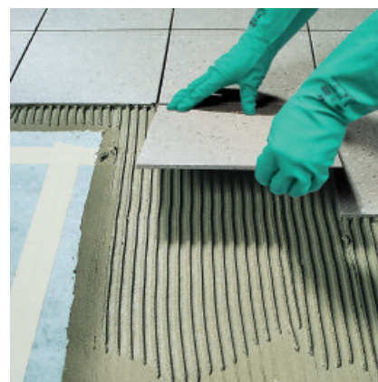
6. ... weitestgehend hohlraumfrei verlegen.
