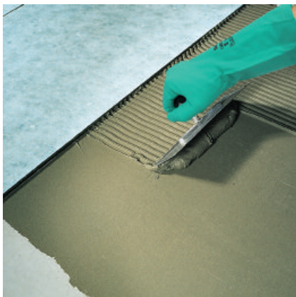
1. Auf den vorbereiteten Untergrund PCI Flexmörtel, PCI Flexmörtel-Schnell, PCI Nanoflott oder PCI Nanoflott light aufkämmen.
