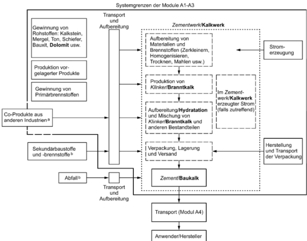
Abbildung 2: Systemgrenzen der Zementproduktion nach ÖNORM EN 16908 [9]
