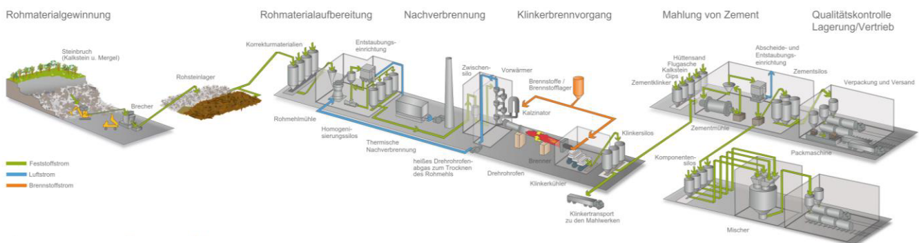
Abbildung 1: Schematische Darstellung des Zementherstellungsprozesses der Alpacem Zement Austria GmbH vom Steinbruch bis zum Versand
